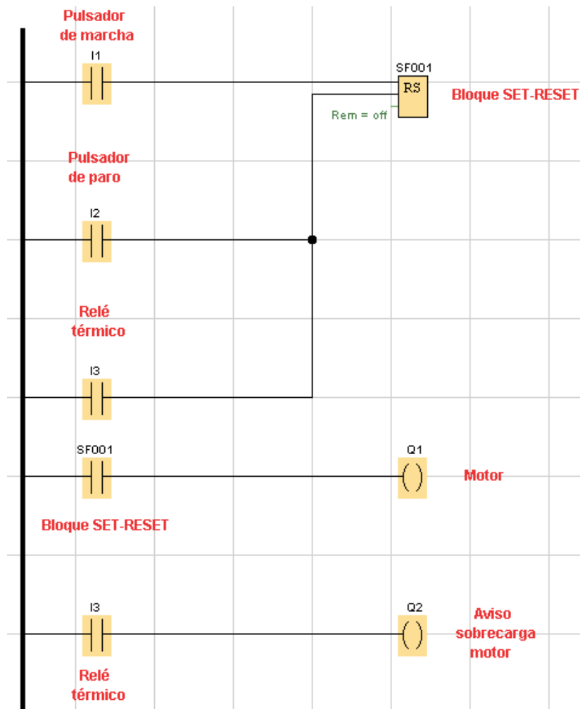
Programación 2: LD (ladder Diagram) o lenguaje de contactos con SET-RESET
