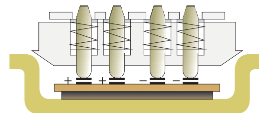
Detalle de conexionado de la salida binaria al carril de datos
