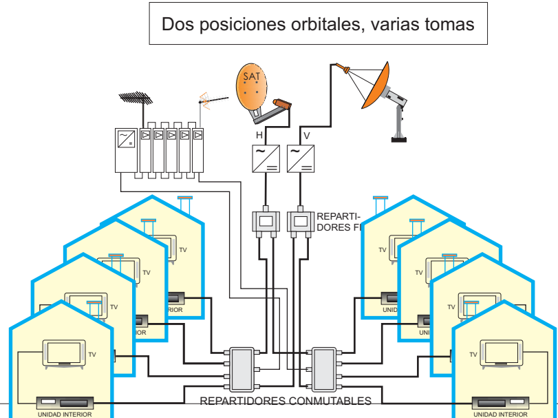
Una Polaridad, varias tomas
