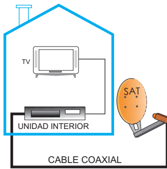
Una polaridad, una toma de usuario.
